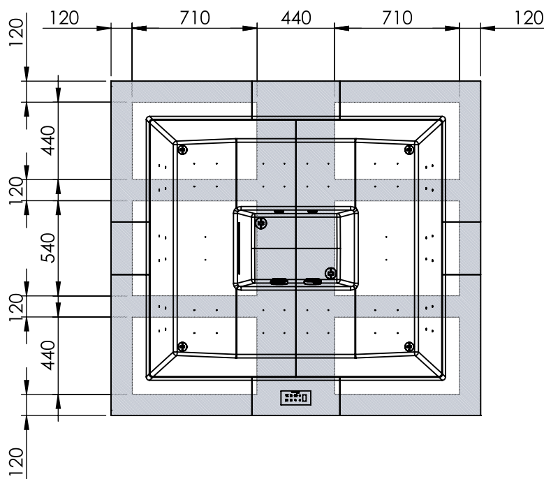
SCHEMA PER EVENTUALI RINFORZI A PAVIMENTO SCHEME FOR FLOOR REINFORCEMENTS
